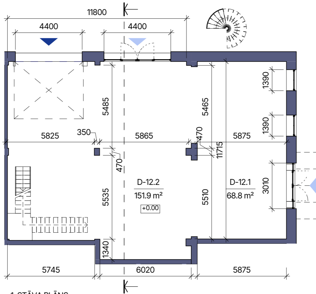
1. STĀVA PLĀNS
