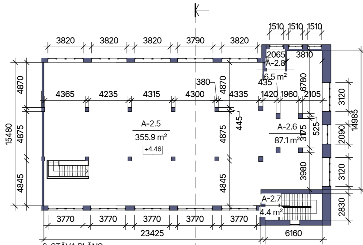
2. STĀVA PLĀNS
