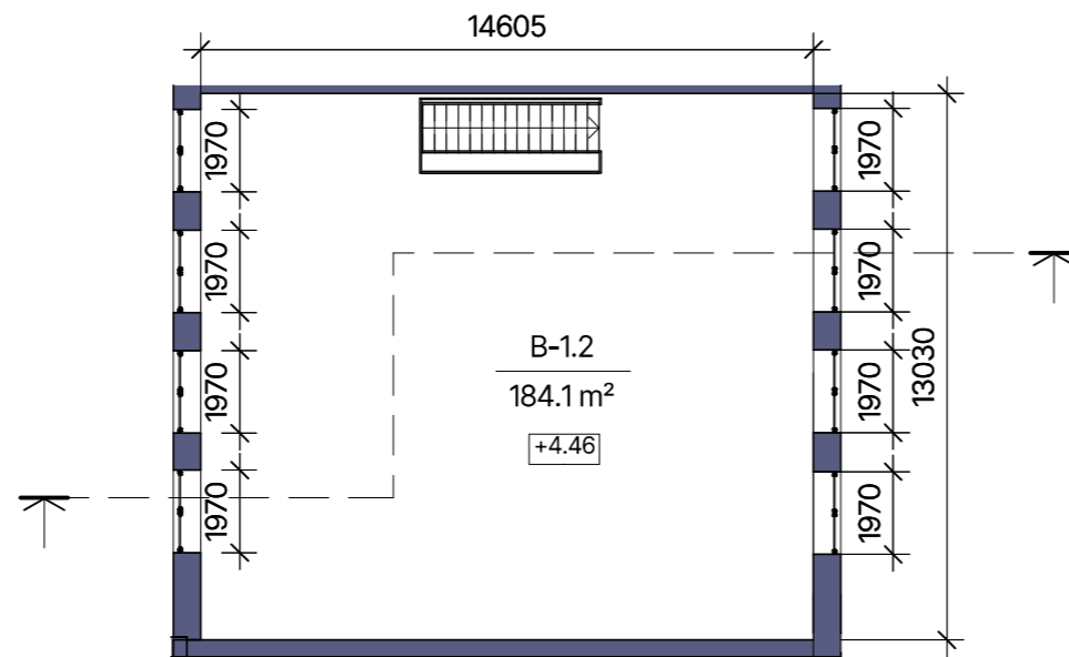
2. STĀVA PLĀNS
