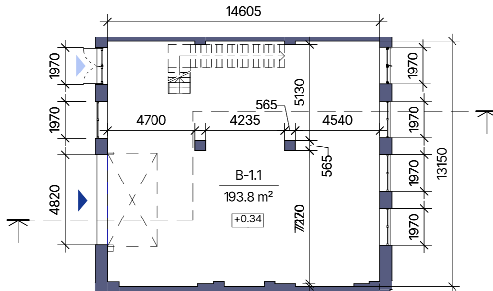
1. STĀVA PLĀNS
