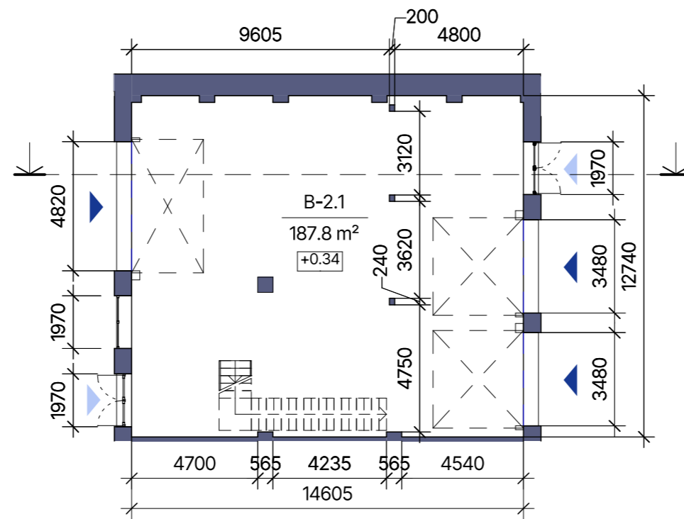
1. STĀVA PLĀNS
