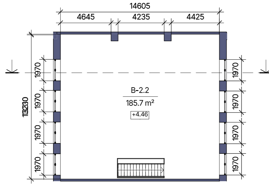
2. STĀVA PLĀNS
