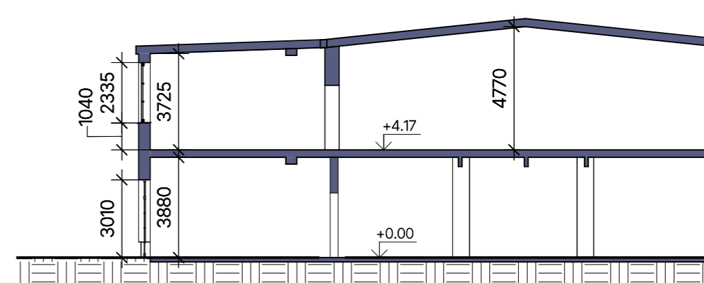
GRIEZUMS
