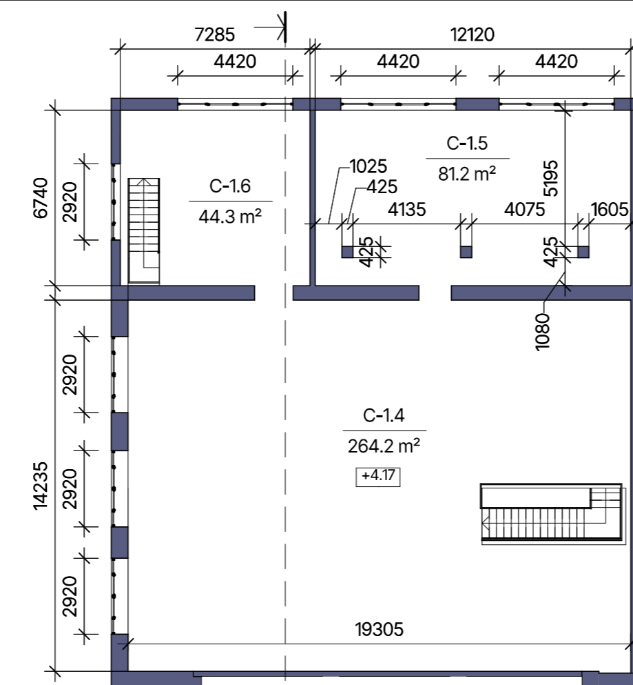
2. STĀVA PLĀNS
