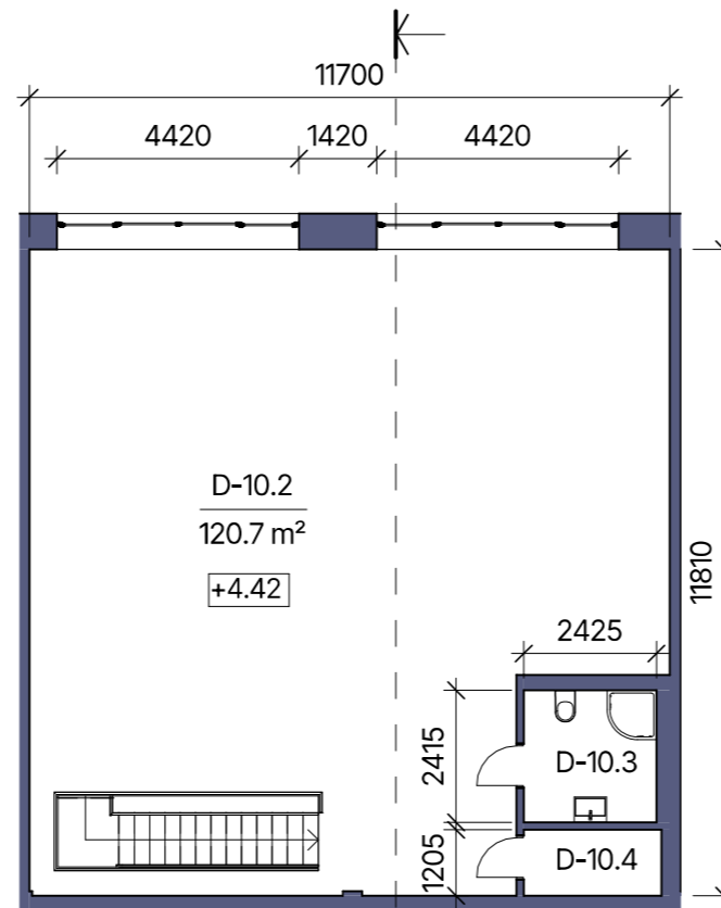
2. STĀVA PLĀNS
