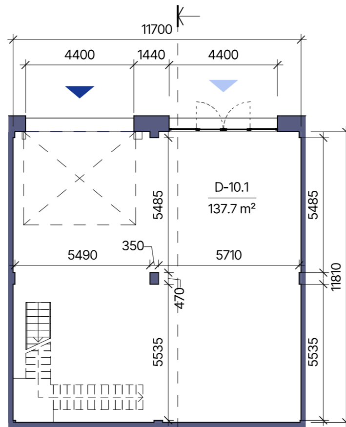
1. STĀVA PLĀNS
