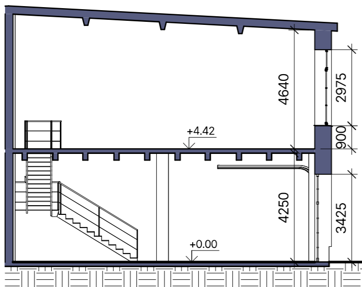
ŠĶĒRSGRIEZUMS
