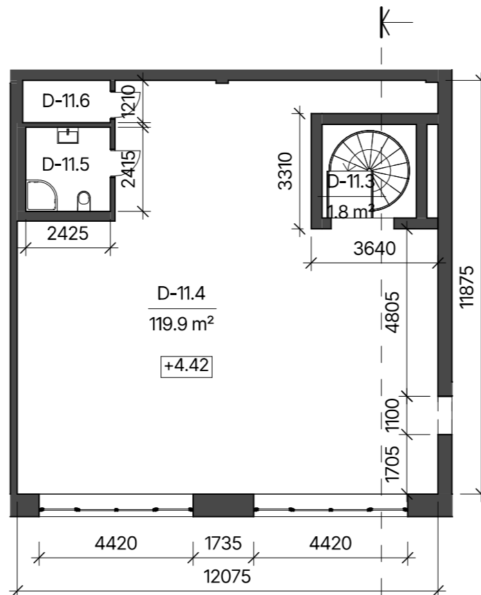
2. STĀVA PLĀNS
