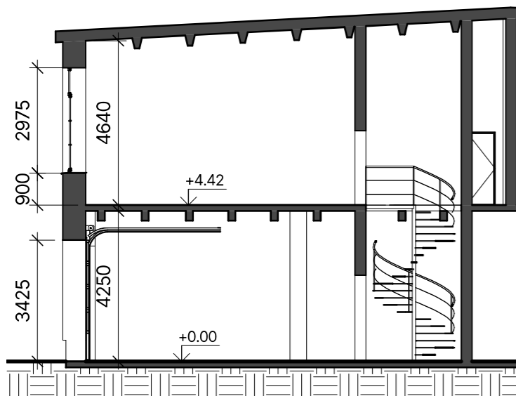
ŠĶĒRSGRIEZUMS
