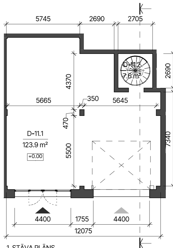
1. STĀVA PLĀNS
