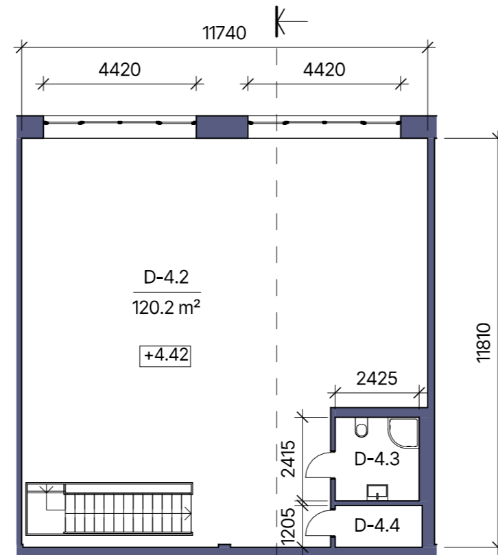
2. STĀVA PLĀNS
