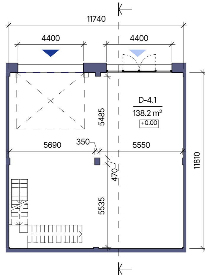
1. STĀVA PLĀNS
