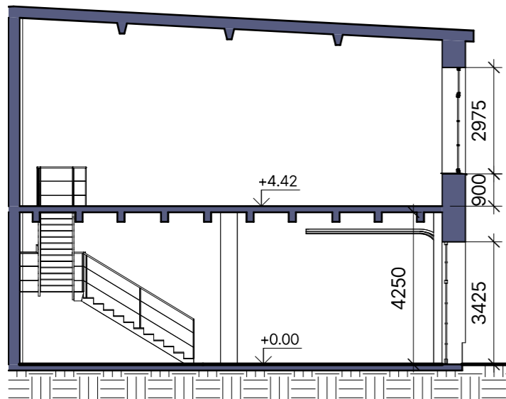
ŠĶĒRSGRIEZUMS
