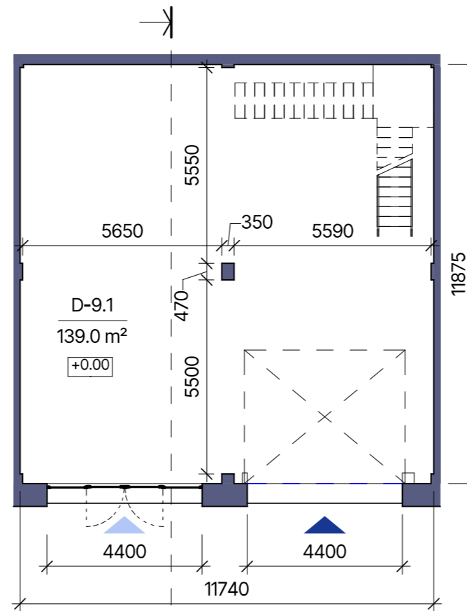
1. STĀVA PLĀNS
