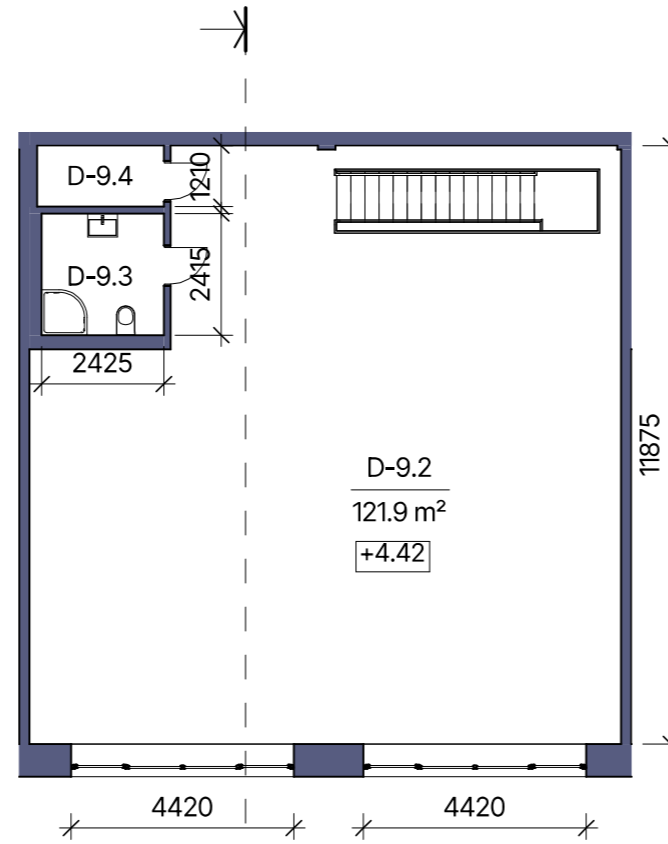
2. STĀVA PLĀNS
