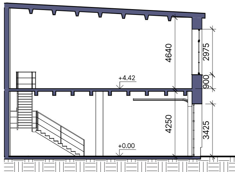
ŠĶĒRSGRIEZUMS
