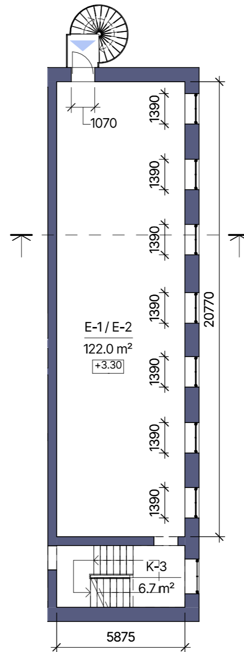
2. STĀVA PLĀNS
